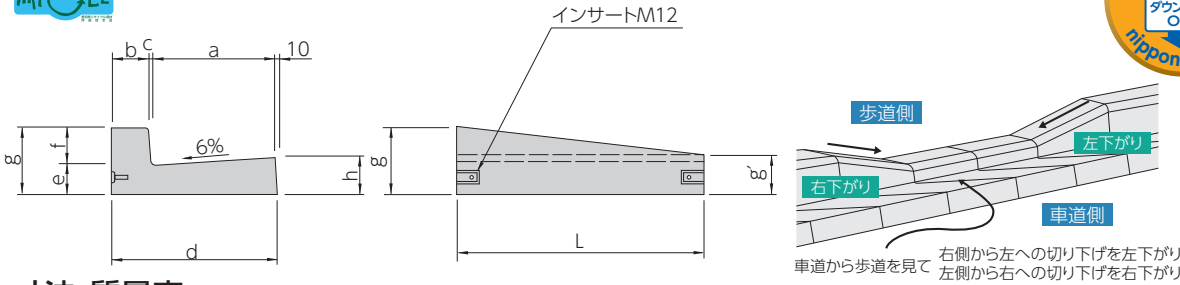
寸法・質量表(単位mm)
