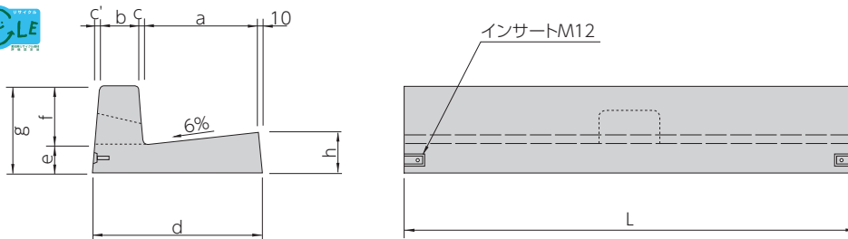
寸法・質量表(単位mm)
