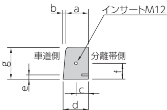
寸法・質量表(単位mm)
