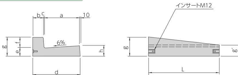
寸法・質量表(単位mm)
